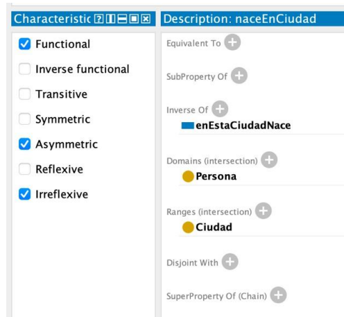
Figura 6. Ontología SCORE. Ejemplo de cardinalidad (1). Fuente: Protégé 5.6.4. Ontologia_score.ofn (elaboración propia).
