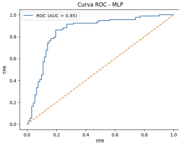
Figura 5: Curva ROC para el modelo MLP ( AUC = 0.85 )
