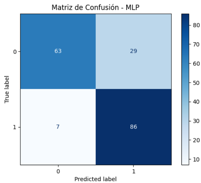
Figura 14: Matriz de confusión del modelo MLP
