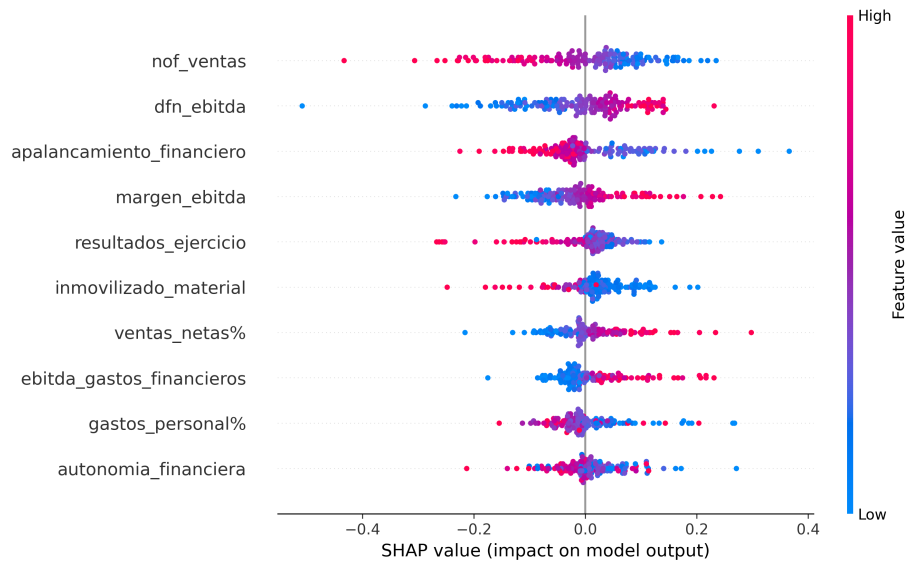
Figura 6: Importancia global de variables (summary plot) – MLP
