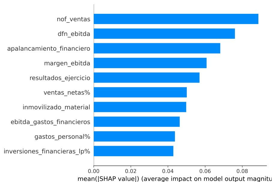
Figura 7: Impacto medio absoluto por variable – MLP
