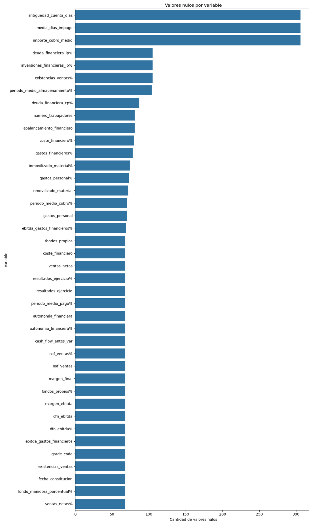
Figura 11: Valores nulos por variable
