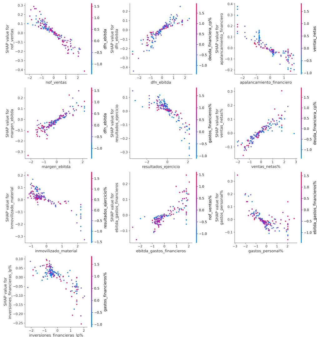
Figura 8: Gráficos de dependencia SHAP para las principales variables – MLP
