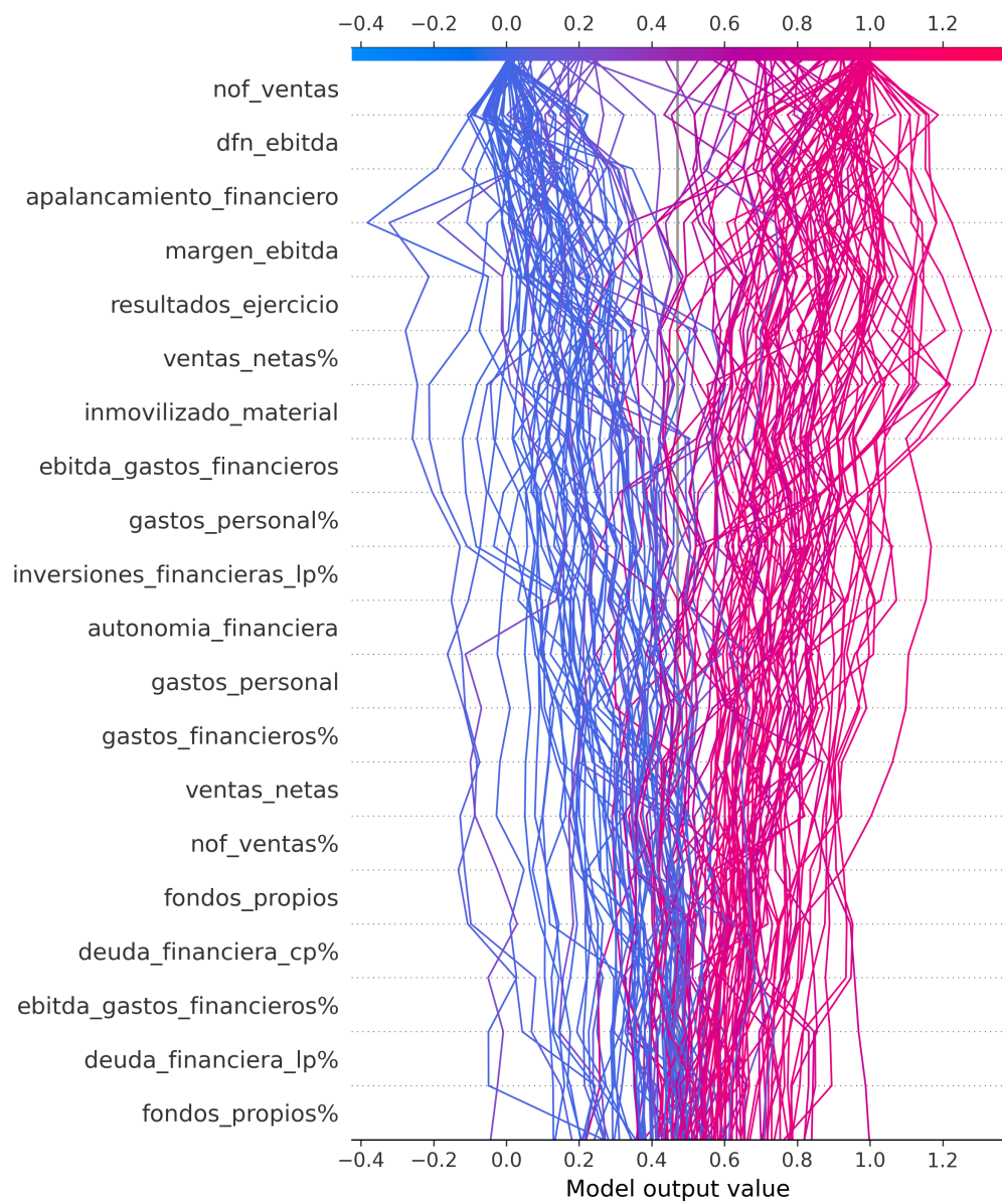
Figura 15: Trayectoria de decisiones (decision plot) – MLP
