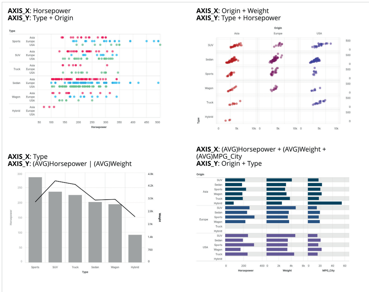
Figura 3. Ejemplos de diferentes composiciones visuales como resultado del uso de diferentes combinaciones de variables y propiedades posicionales
