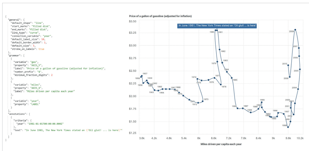
Figura 1. Especificación gramatical de un diagrama de dispersión conectado en SCImago Graphica
