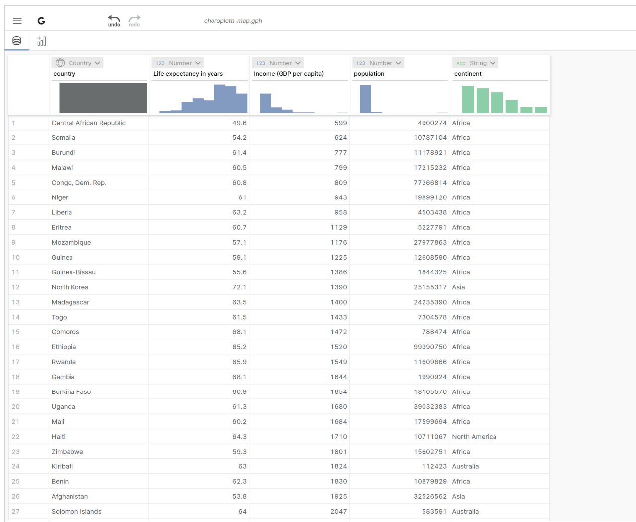
Figura 6. Pantalla inicial de SCImago Graphica después de cargar los datos
