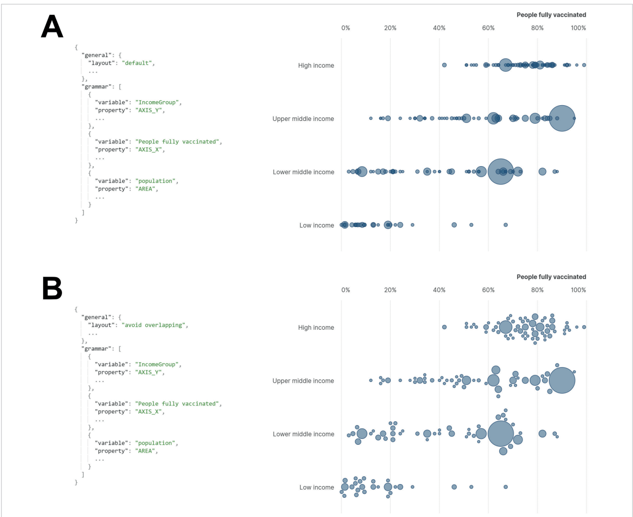
Figura 5. A) Ejemplo de composición visual por propiedades posicionales. B) Ejemplo de composición visual combinando propiedades posicionales con un algoritmo que evita la superposición. La posición Y de cada símbolo viene dada por la variable categórica "IncomeGroup" y por la aplicación del algoritmo, mientras que la posición X viene dada exclusivamente por la variable cuantitativa "People fully vaccinated".
