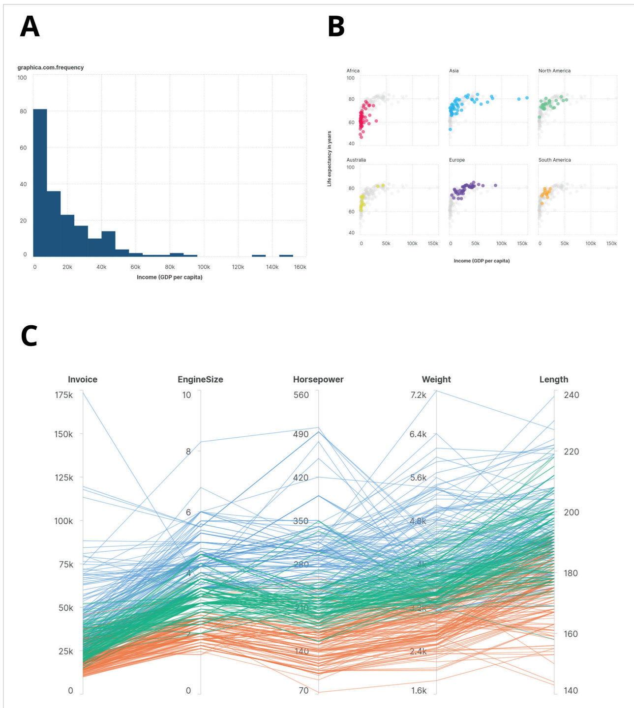
Figura 8. A) Histograma. B) Múltiples pequeños. C) Coordenadas paralelas
