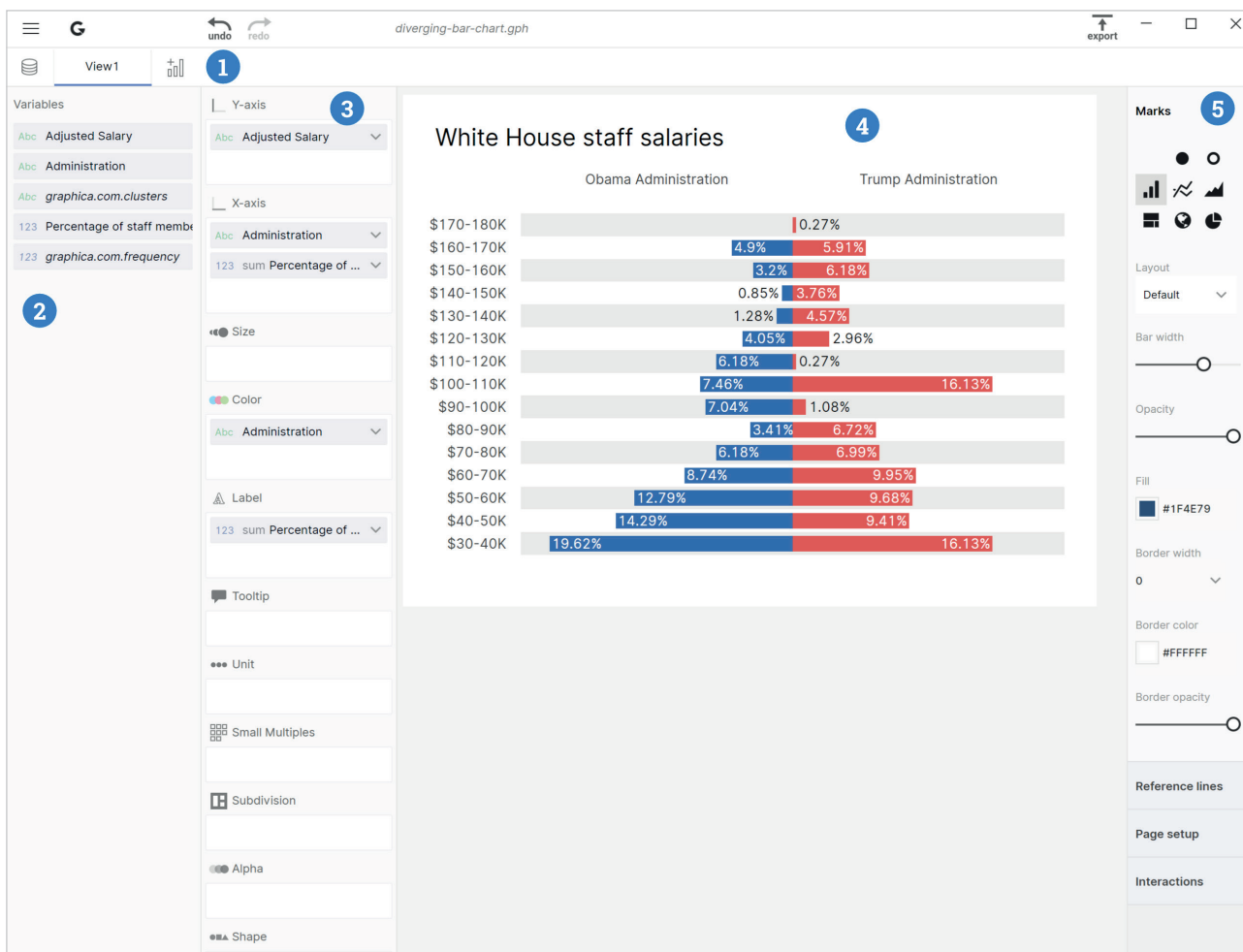
Figura 7. Interfaz SCImago Graphica para visualización de datos mediante mapeo visual
