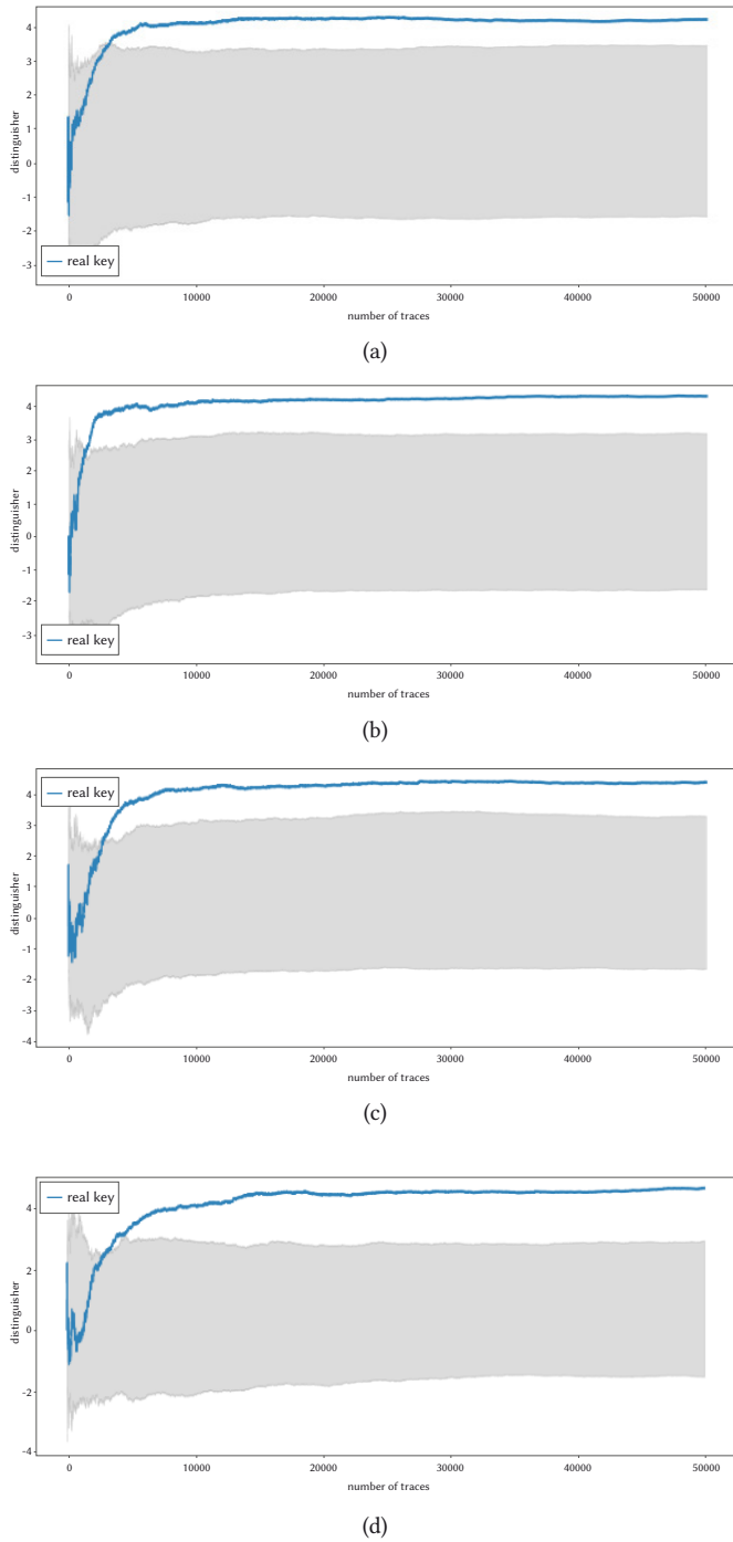
Fig. 12. Attack result of \delta_{1,0} : (a) Byte 3 (b) Byte 2 (c) Byte 1 (d) Byte 0.
