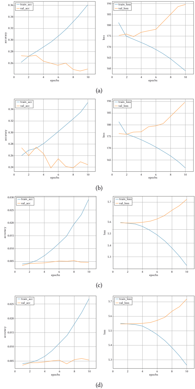
Fig. 13. Training result of a_0 : (a) Byte 3 (b) Byte 2 (c) Byte 1 (d) Byte 0.
