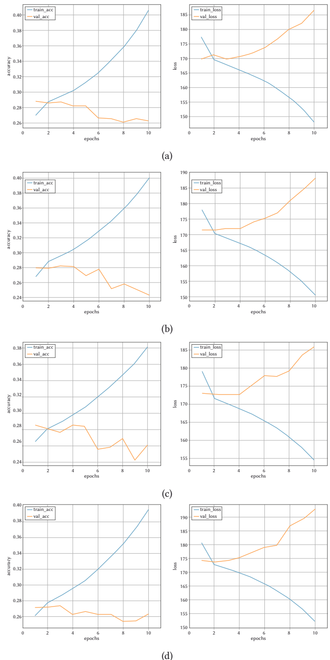
Fig. 11. Training result of \delta_{1,0} : (a) Byte3 (b) Byte 2 (c) Byte 1 (d) Byte 0.
