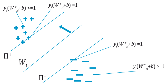
Fig. 7. Margin Hyperplane.
